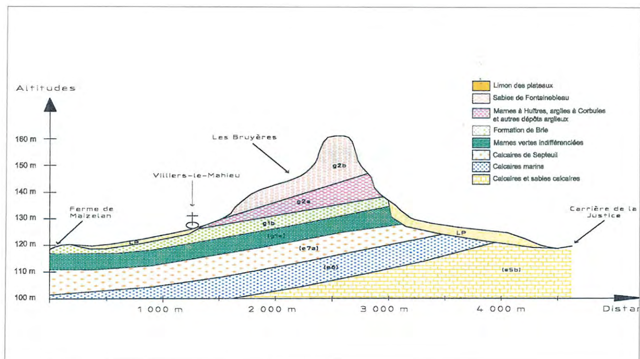
Coupe géologique simplifiée de la commune de Villiers-le-Mahieu, extrait de l'étude du schéma directeur de l'eau, bureau d'étude V. Ruby, janvier 2001
